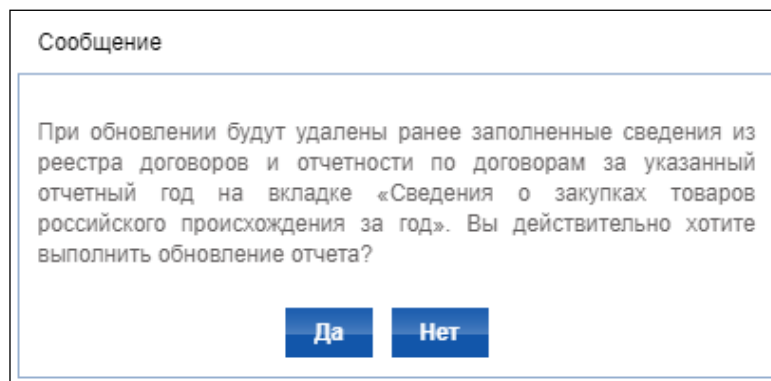
Рисунок 23. Информационное сообщение
