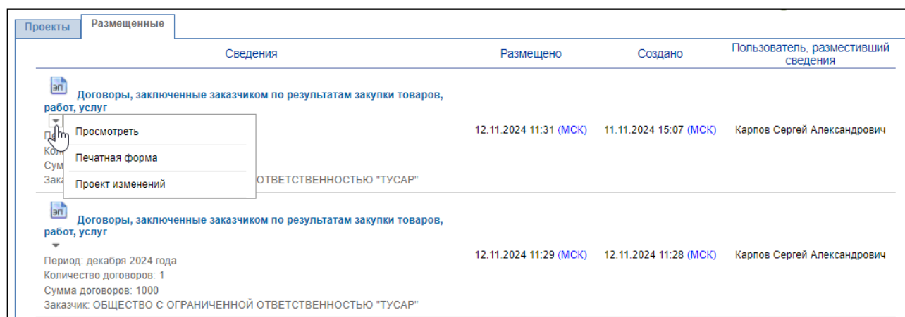
Рисунок 35. Контекстное меню
