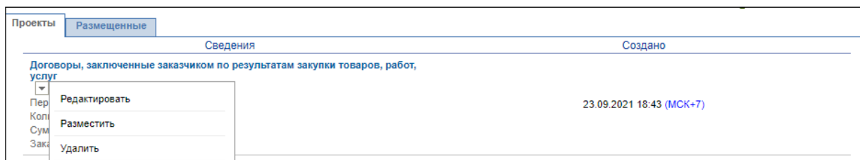
Рисунок 33. Контекстно меню
