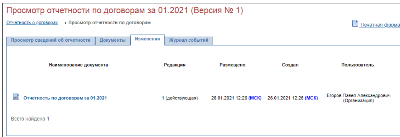
Рисунок 39. Вкладка «Изменения»
