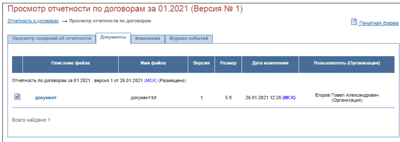
Рисунок 38. Вкладка «Документы»
