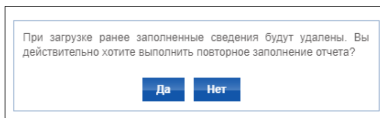
Рисунок 13. Информационное сообщение
